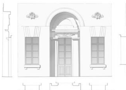
Фрагмент восточного фасада. 1:10
